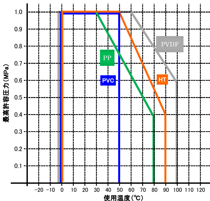
図-4 使用温度と最高許容圧力の関係
