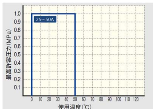
図-2 使用温度と最高許容圧力の関係
