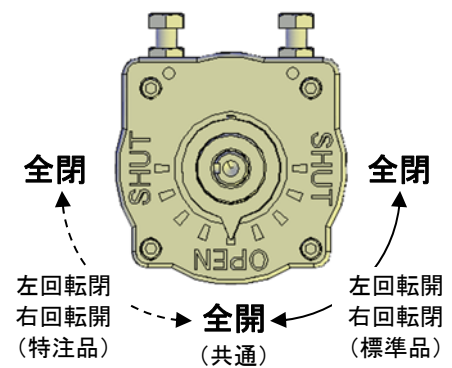
図-4 キャップ式のインジケータ動作
