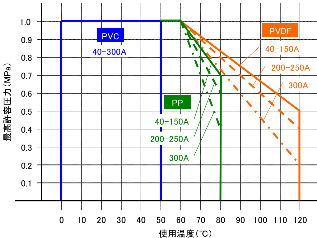
図-4 使用温度と最高許容圧力の関係
