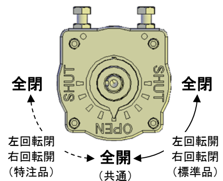
図-6 ハンドル式のインジケータ動作
