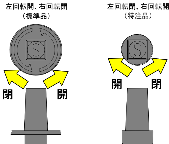
図-3 キャップ式のキャップ操作
