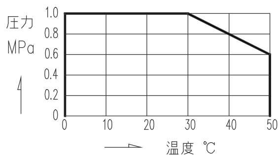
図-6 使用温度と最高許容圧力の関係
