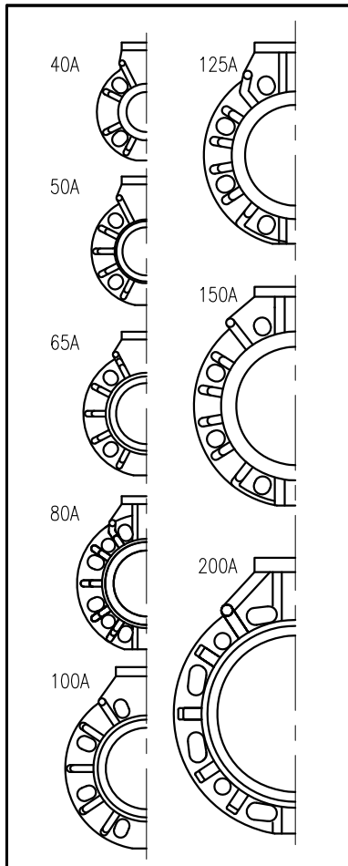
寸法表
